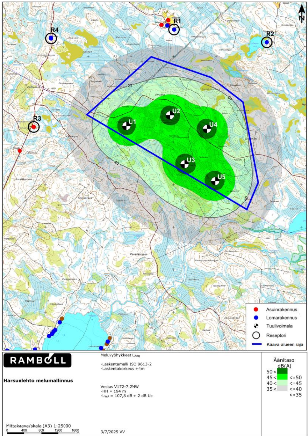
Kuva 72. Harsunlehdon tuulivoimapaiston melumallinnus ja kaavaluonnoksen 2025 aluerajaus.
