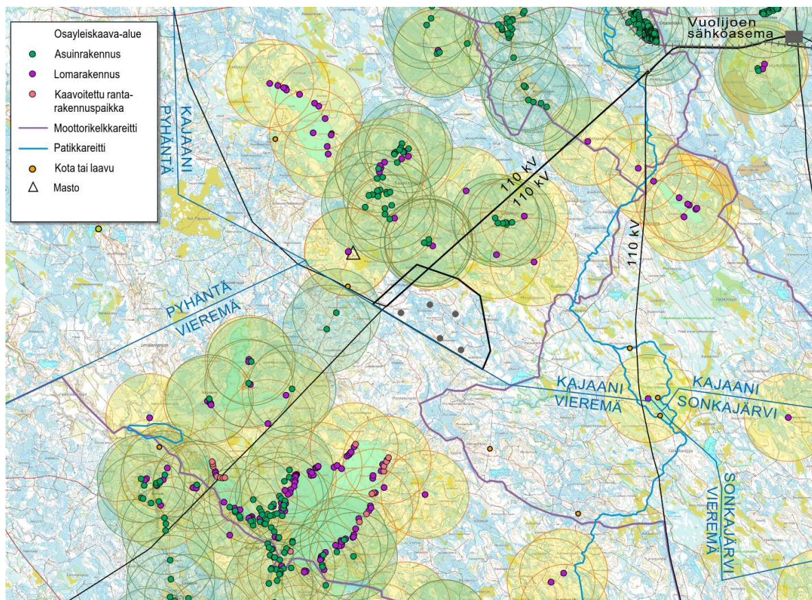
Kuva 36. Osayleiskaava-alueen ja sen lähiympäristön nykyinen maankäyttö (huomioitu myös myönnetty rakennus-, ympäristö- ja maa-ainesluvut). Tuulipuistoaluetta lähimpien asuin- ja lomarakennusten ympärille on piirretty säteeltään 1,5 km oleva raja, jota käytettiin tuulivoimaloiden alustavassa sijoitussuunnittelussa vähimmäisetäisyytenä asutuksen ja voimaloiden välillä. Kaavaluonnoksen voimaloiden sijoitussuunnittelussa on käytetty kaupungin tuulivoimaohjelman mukaista 2 km vähimmäisetäisyyttä asutukseen ja loma-asutukseen.
